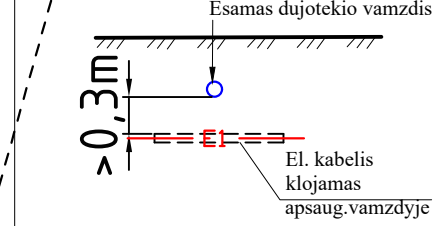
Dujotekio ir projektuojamų elektros kabelių susikirtimų pjūvis
