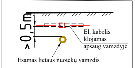
Lietaus ir projektuojamų elektros kabelių susikirtimų pjūvis
