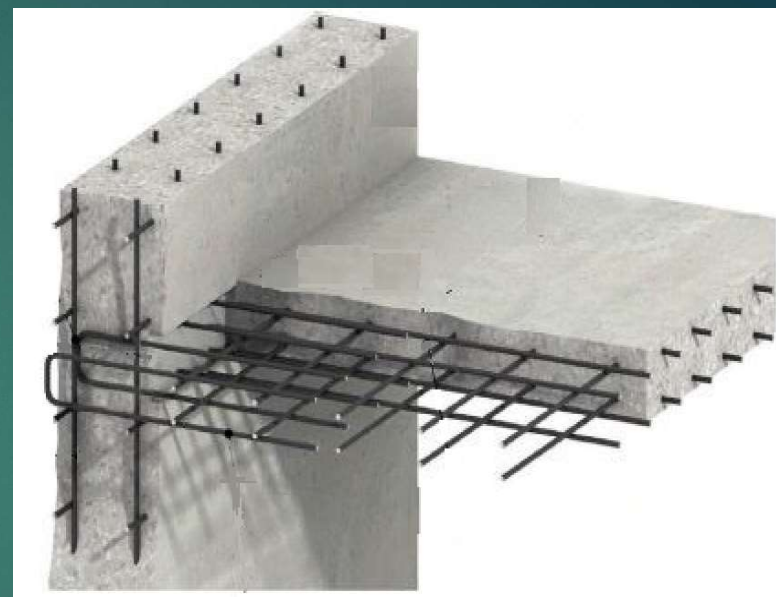
Pav. Betoninės sienos jungtis su perdanga
