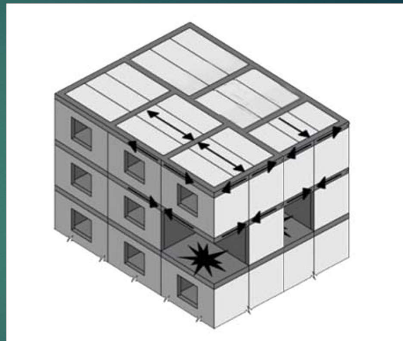
Pav. Laikančios konstrukcijos prasilenkia
