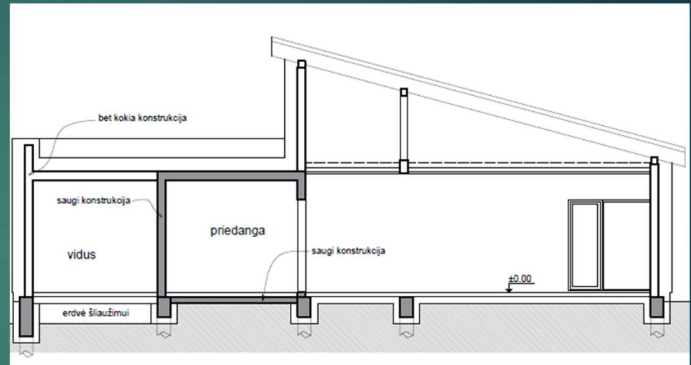
Pav. priedangos vieta individualiame name (pjūvis)
