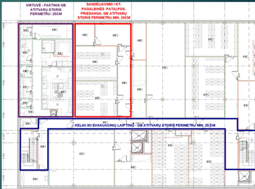
Pav. Priedanga įrengiama rūsyje, tarp betoninių sienų
